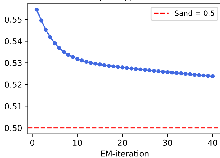
\gamma — type 1
