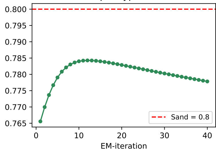
\gamma — type 2
