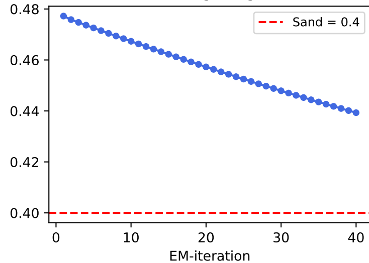
Blandingsvægt \pi
